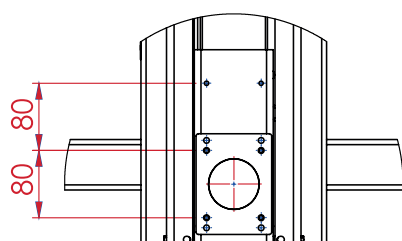
DÉTAIL A
